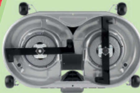
◀ Ontwerp asynchroon maaidek
